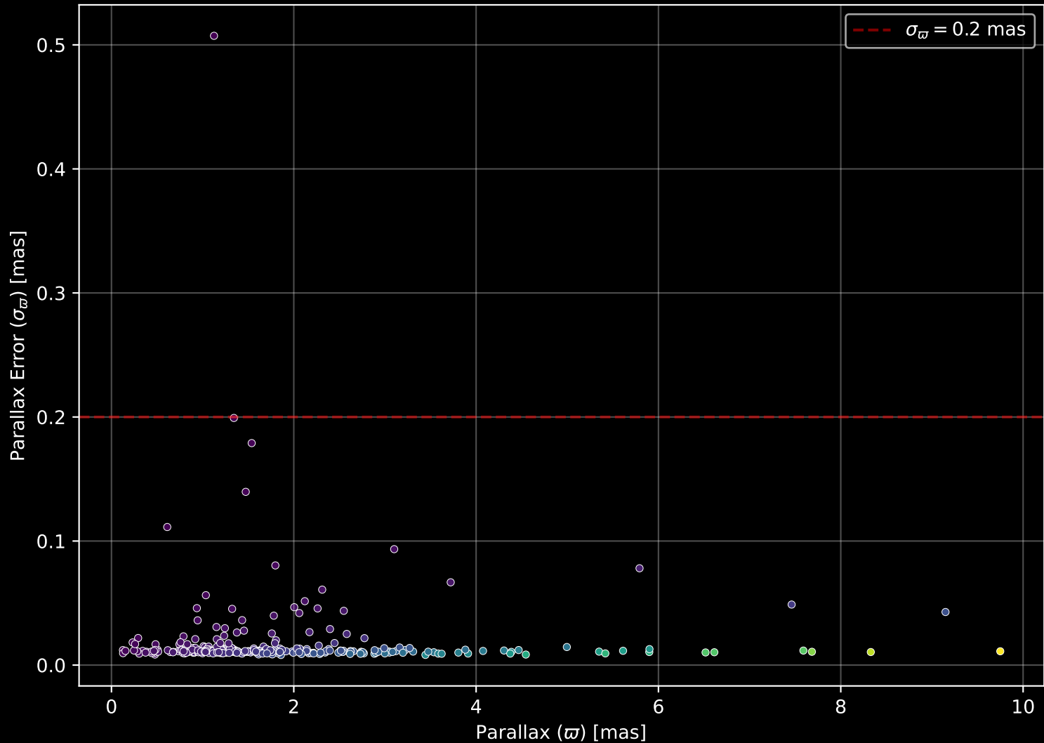
GALAH DR4 Field: [626] Parallax Quality (n= 315)
