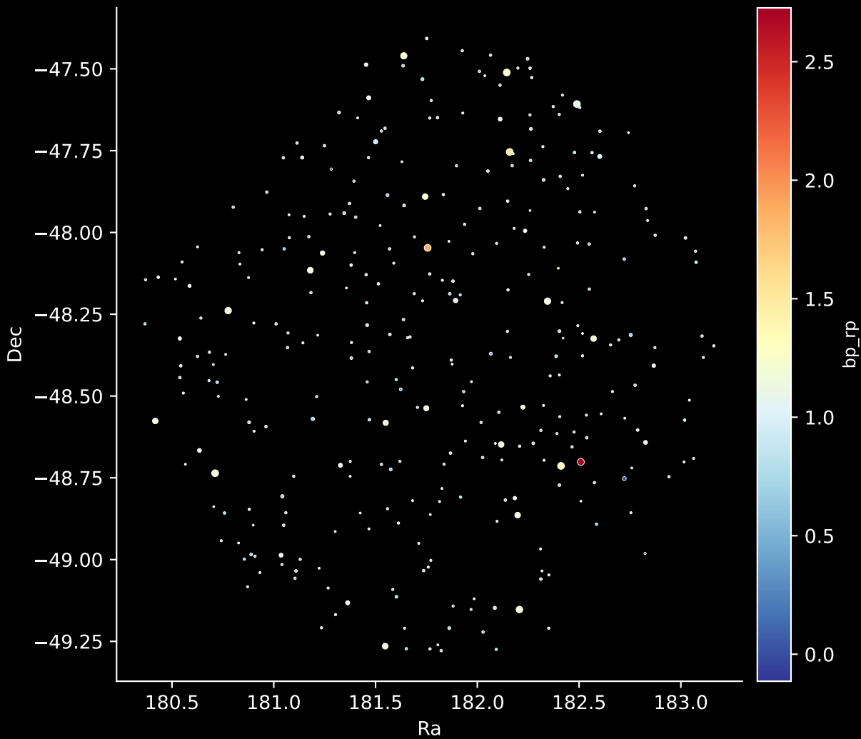
GALAH DR4 Field: [626] Stars: 315
