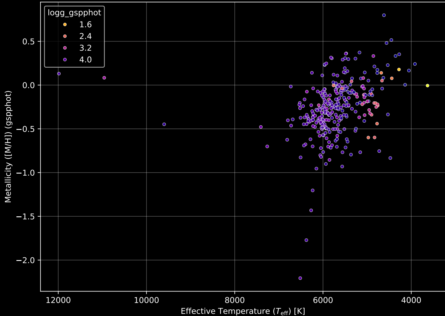
GALAH DR4 Field: [626] Stellar Population Parameters (n= 315)
