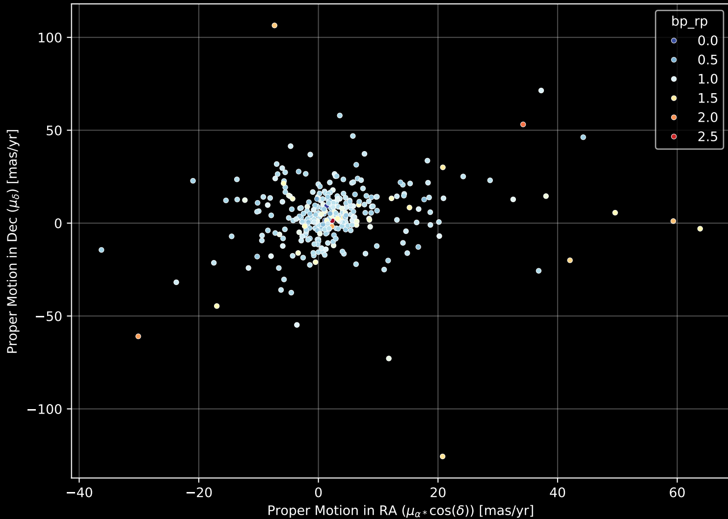
GALAH DR4 Field: [626] Proper Motion Diagram (n= 315)
