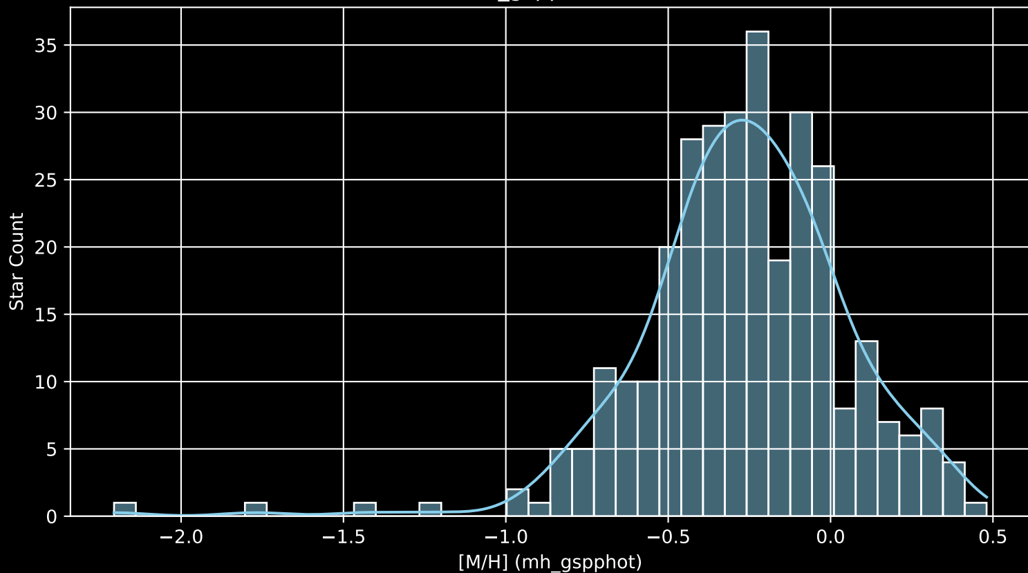
GALAH DR4 Field: [626] [M/H] (mh_gspphot) (n= 313)
